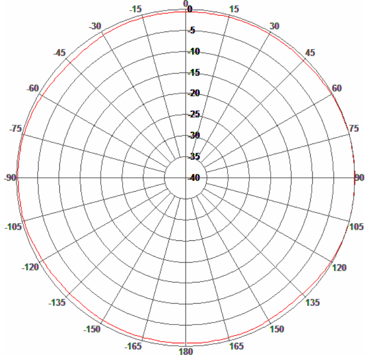
H-Plane Patterns
