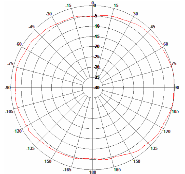
H-Plane Pattern
